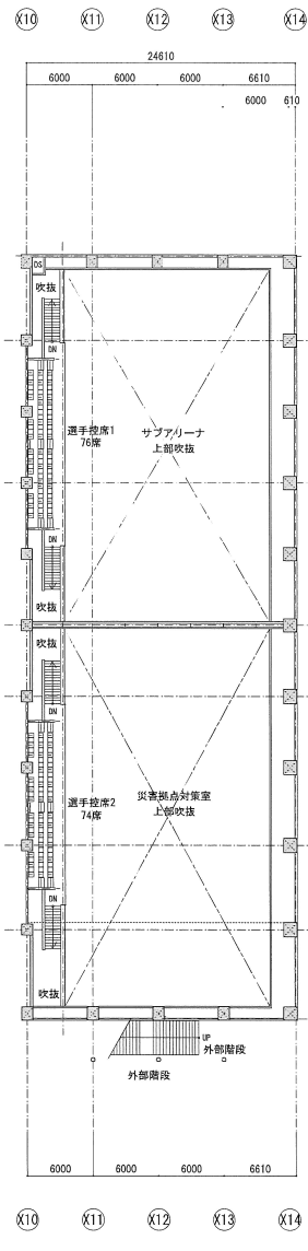
中2階平面図 S=1/250
