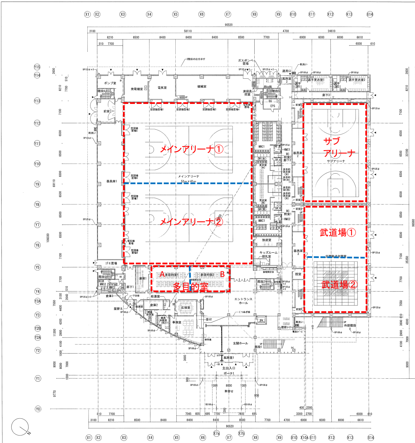
1階平面図 S=1/250
